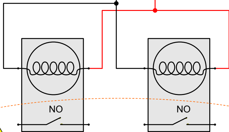
Contacteur de charge 125Vac @ 20A
